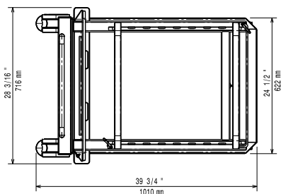
Boven aanzicht
